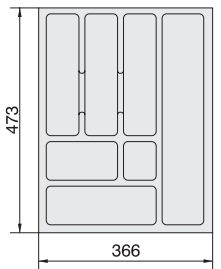
TANDEMBOX 45
