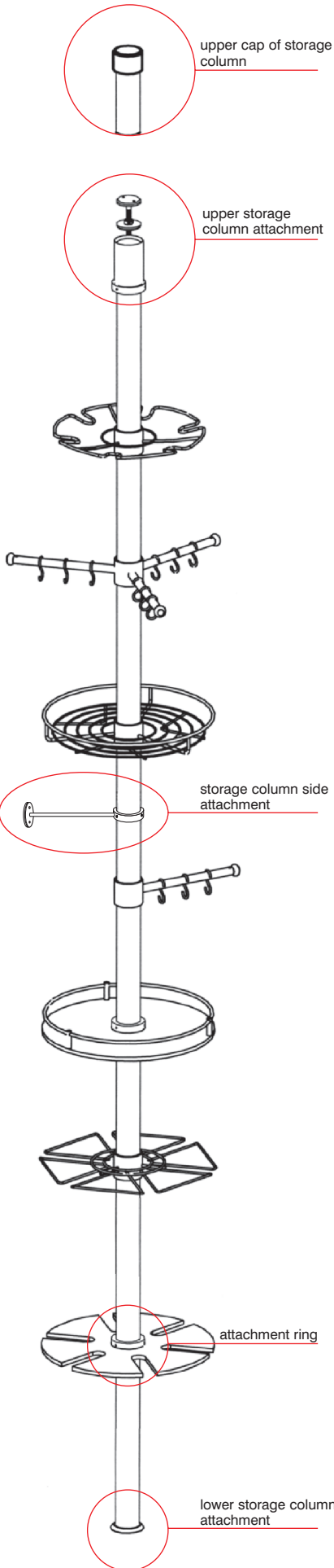
column rod
