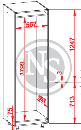
DL/NT180-60/207-P/P
