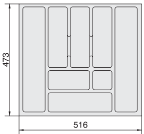
TANDEMBOX 60
